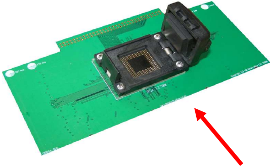
Adaptateur BGA 256 broches pas de 1.27mm
